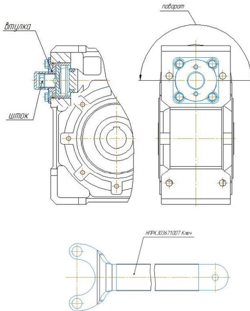
Рисунок 28 - Выборку осевого люфта червячного вала редуктора
