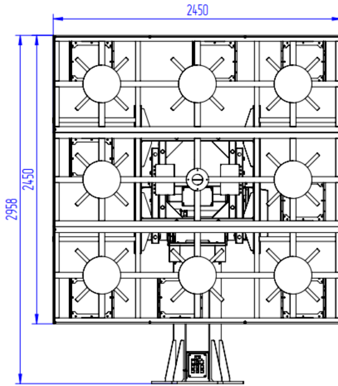
Рисунок 3- Габаритные размеры антенного поста UHF-диапазона
