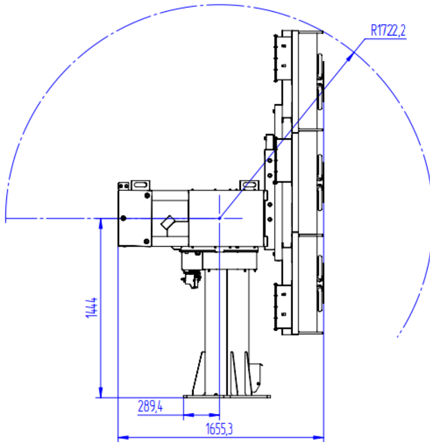
Рисунок 3- Габаритные размеры антенного поста UHF-диапазона
