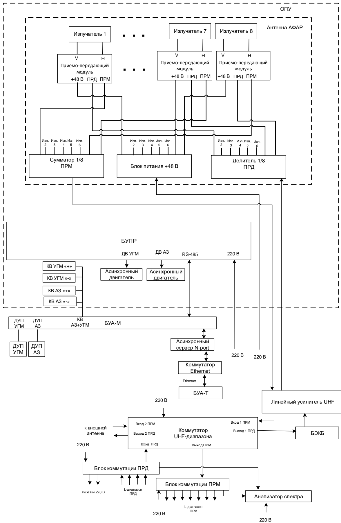
Рисунок 2 - Функциональная схема ППК УНФ
