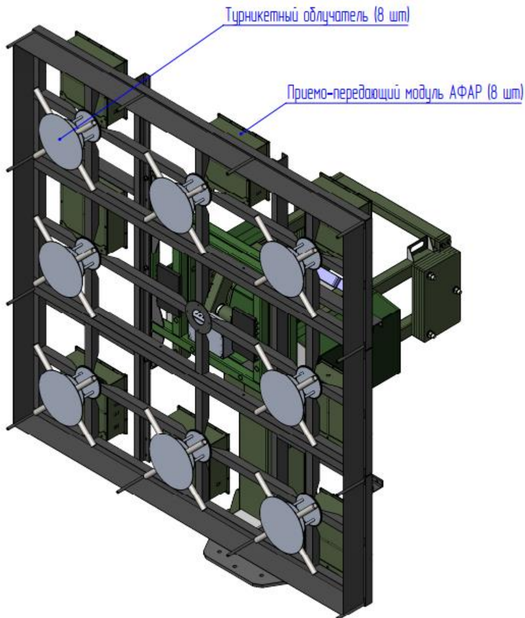
Рисунок 1 Внешний вид ППК UHF
