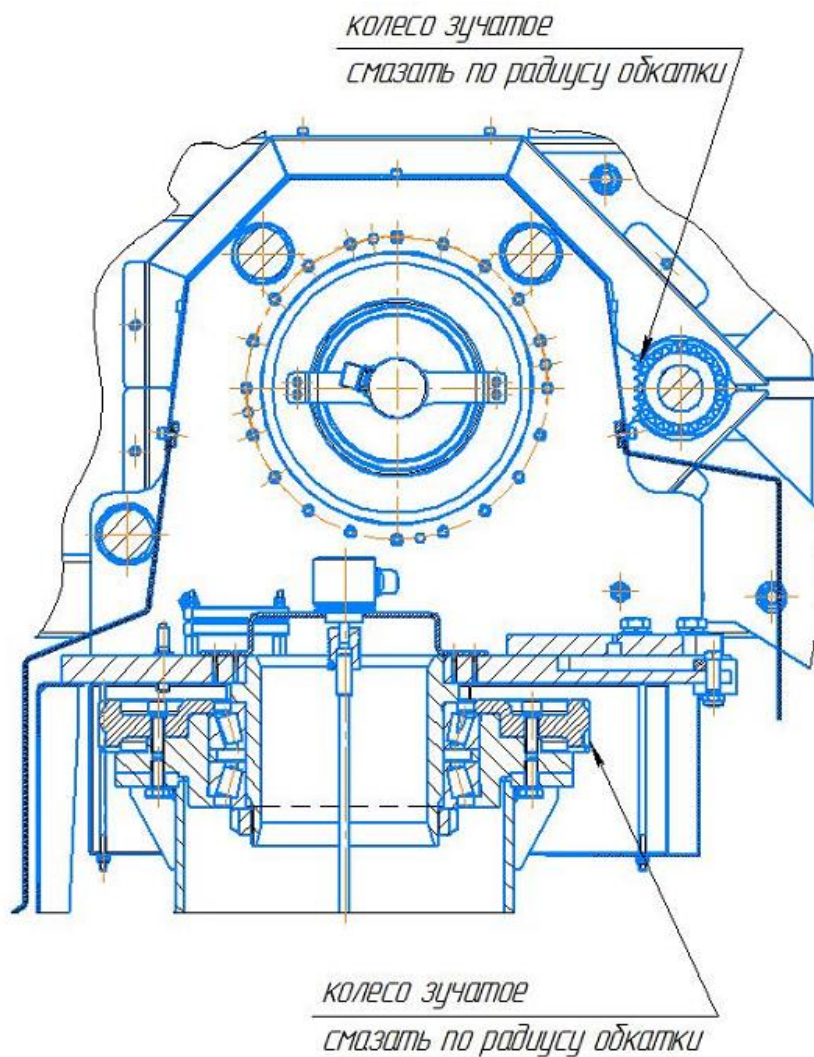
Рисунок 30 - Зубчатые соединения ОПУ
