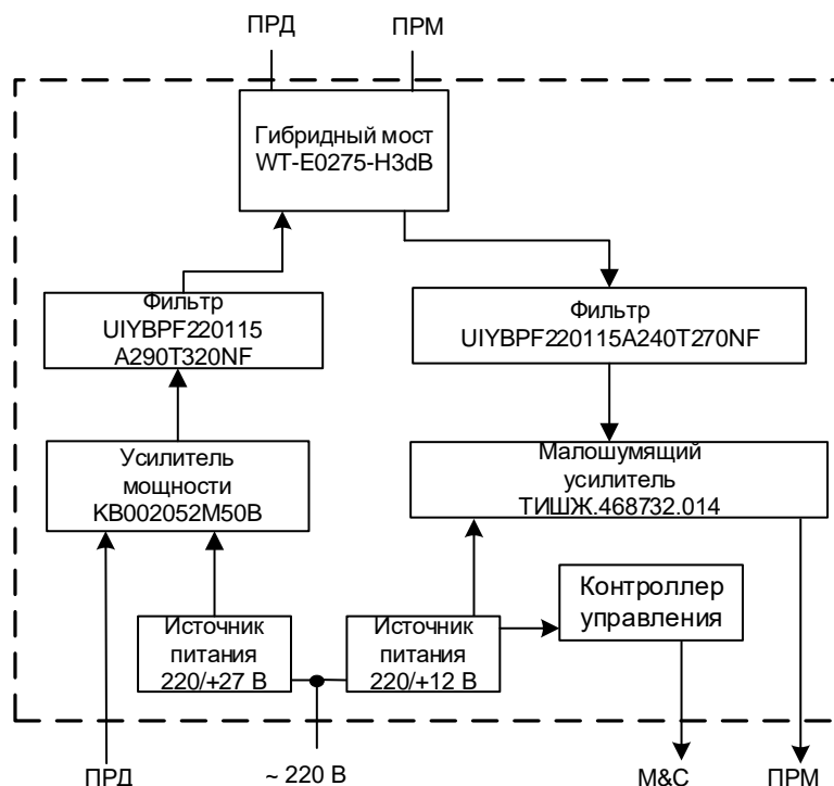
Рисунок 18 – Функциональная схема приема-передающего модуля
