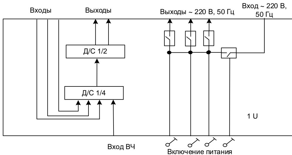
Рисунок 22 - Функциональная схема блока коммутации ПРД
