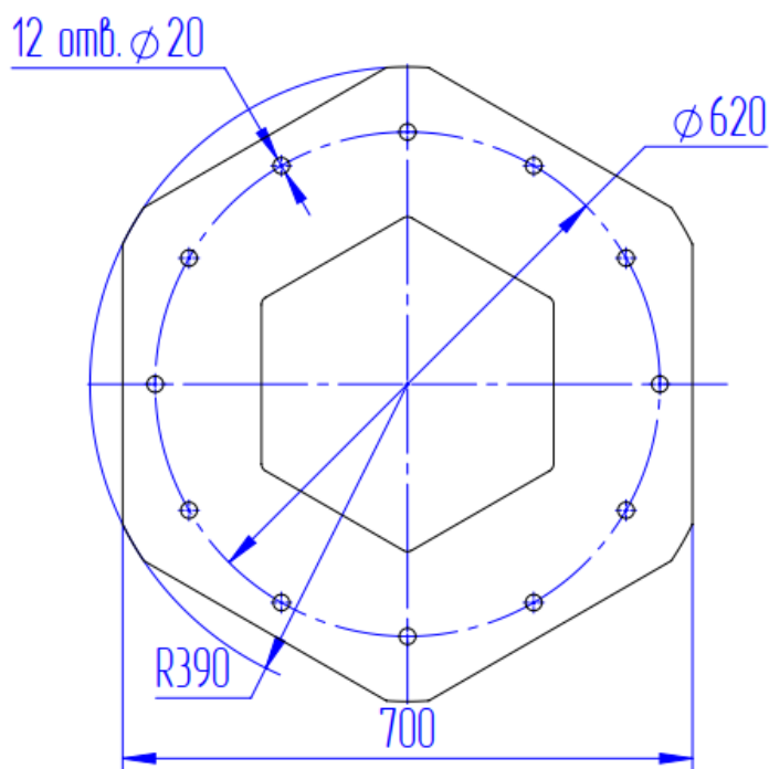
Рисунок 27 - Габаритные размеры переходного фланца ОПУ.
