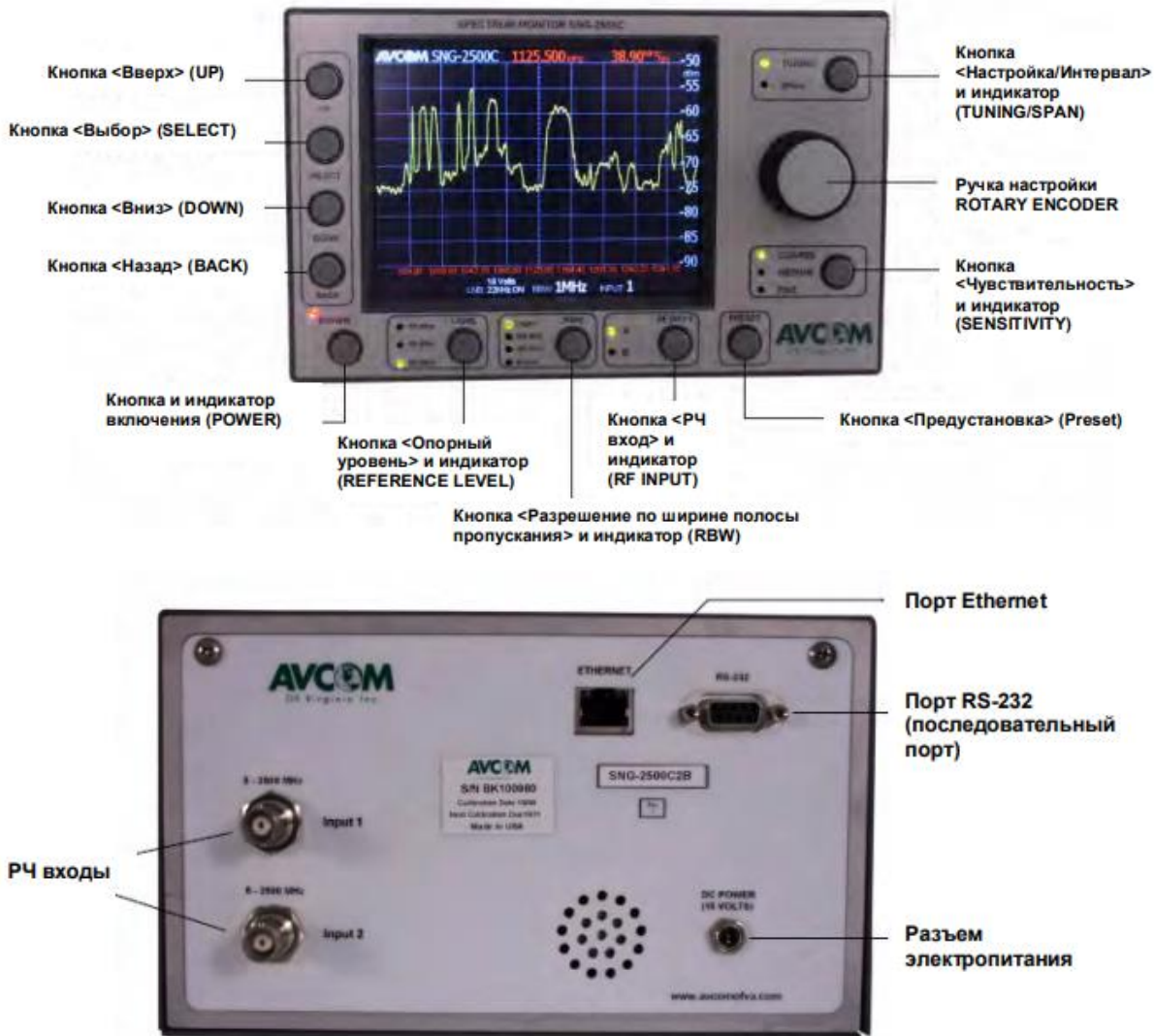
Рисунок 26 – Описание элементов контроля на передней панели и разъемов на задней панели SNG 2500C2NE
